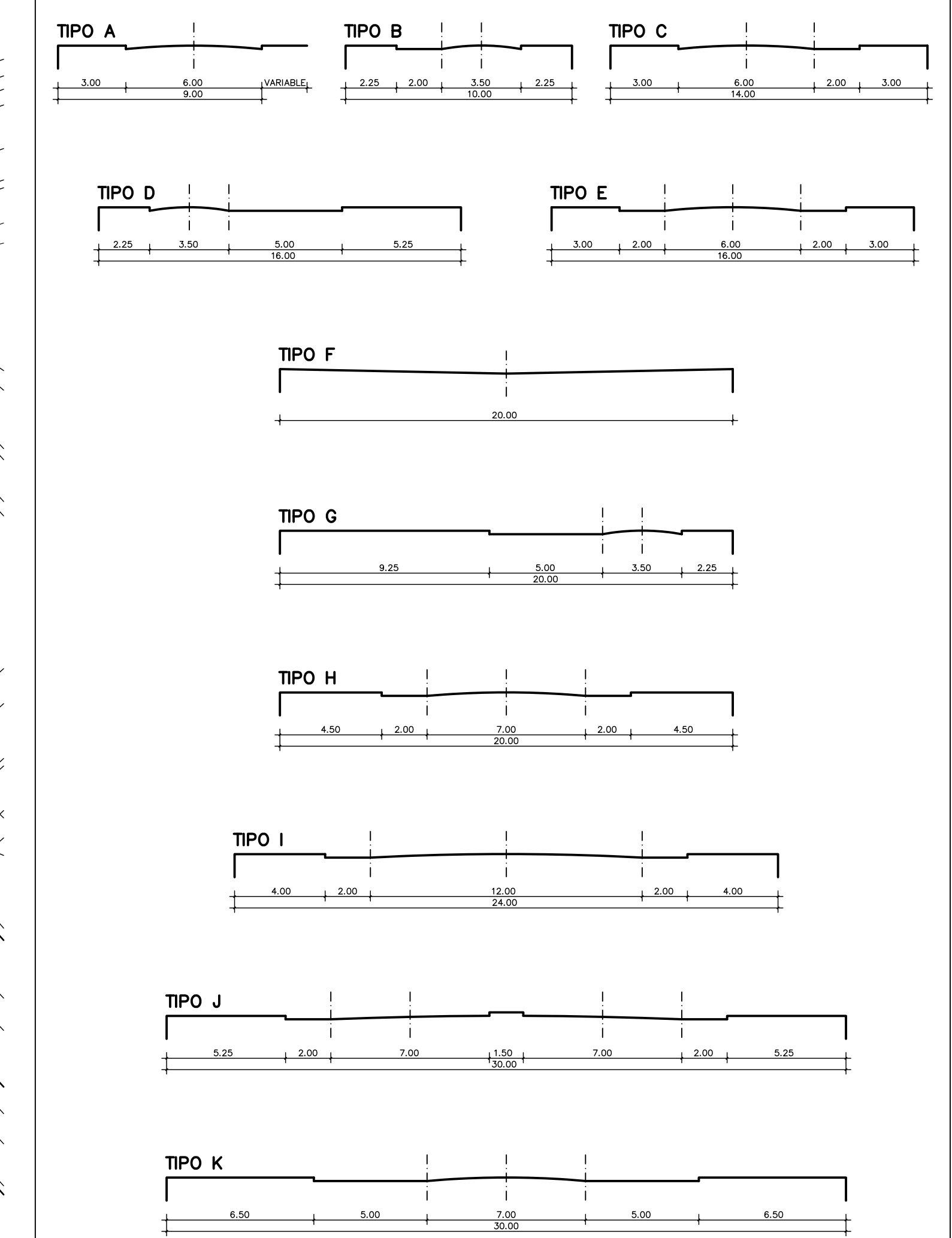
RED VIARIA: SECCIONES TRANSVERSALES TIPO
