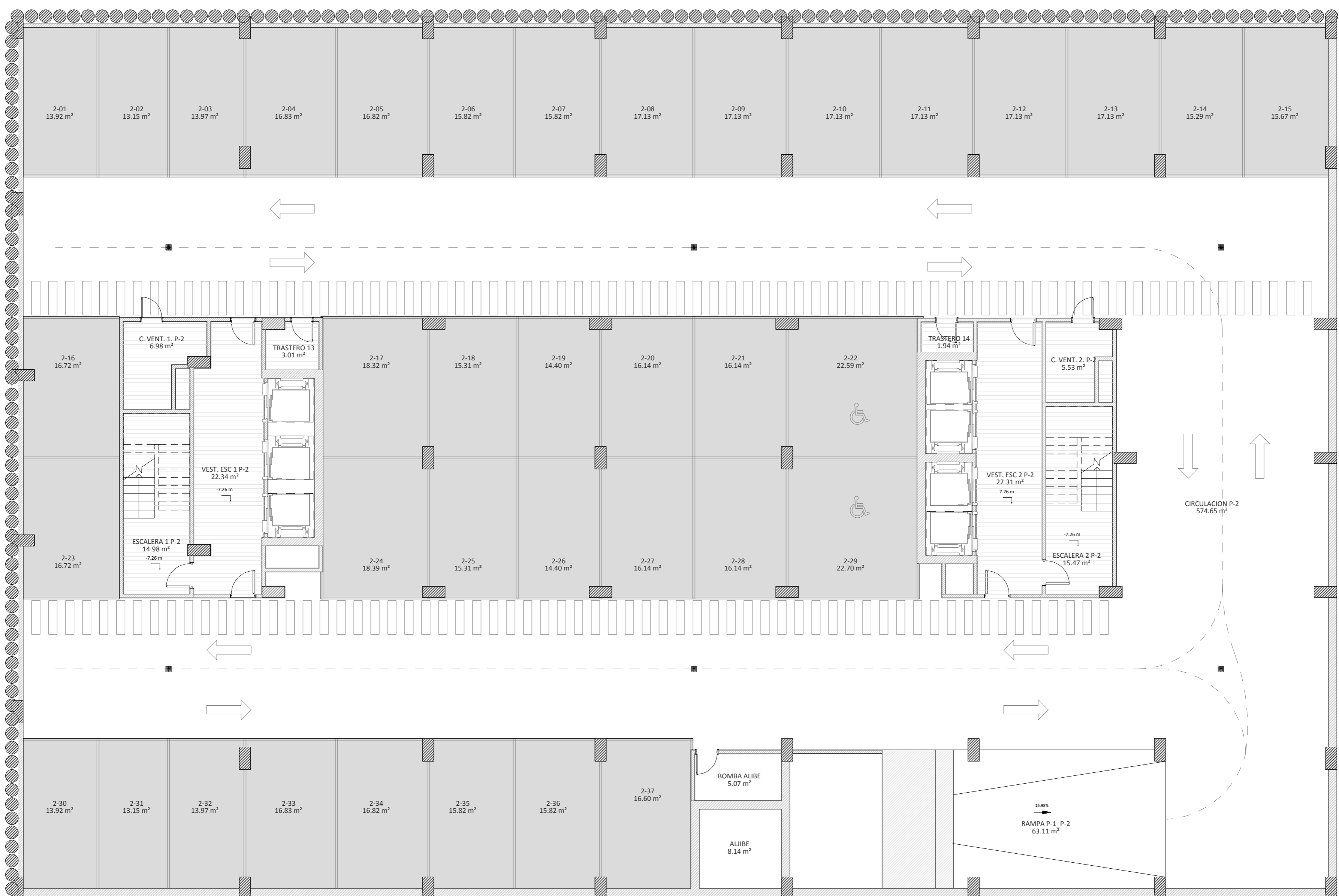
PLANTA SÓTANO -2. 37 PLAZAS APARCAMIENTO
