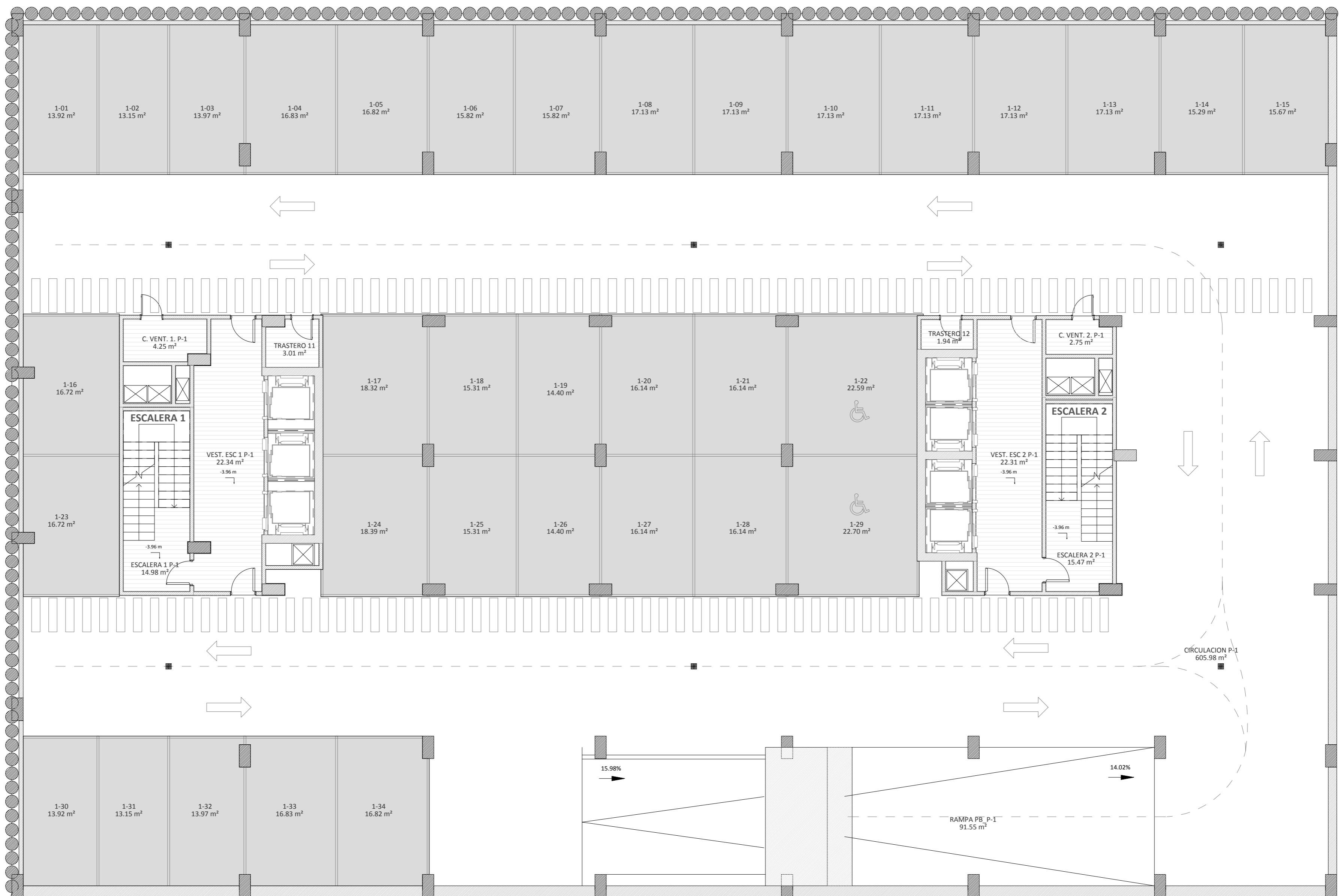
PLANTA SÓTANO -1. 34 PLAZAS APARCAMIENTO
