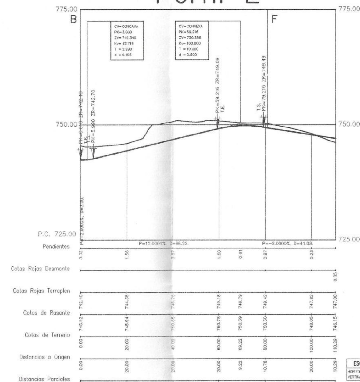
Perfil E
