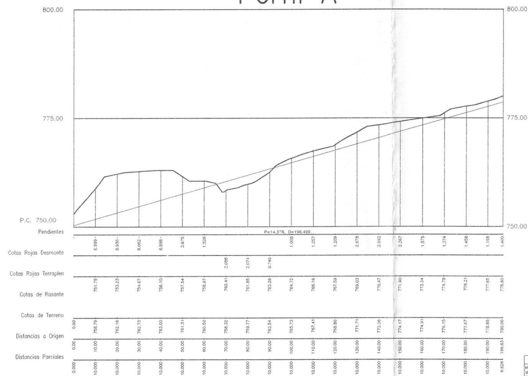
Perfil A
