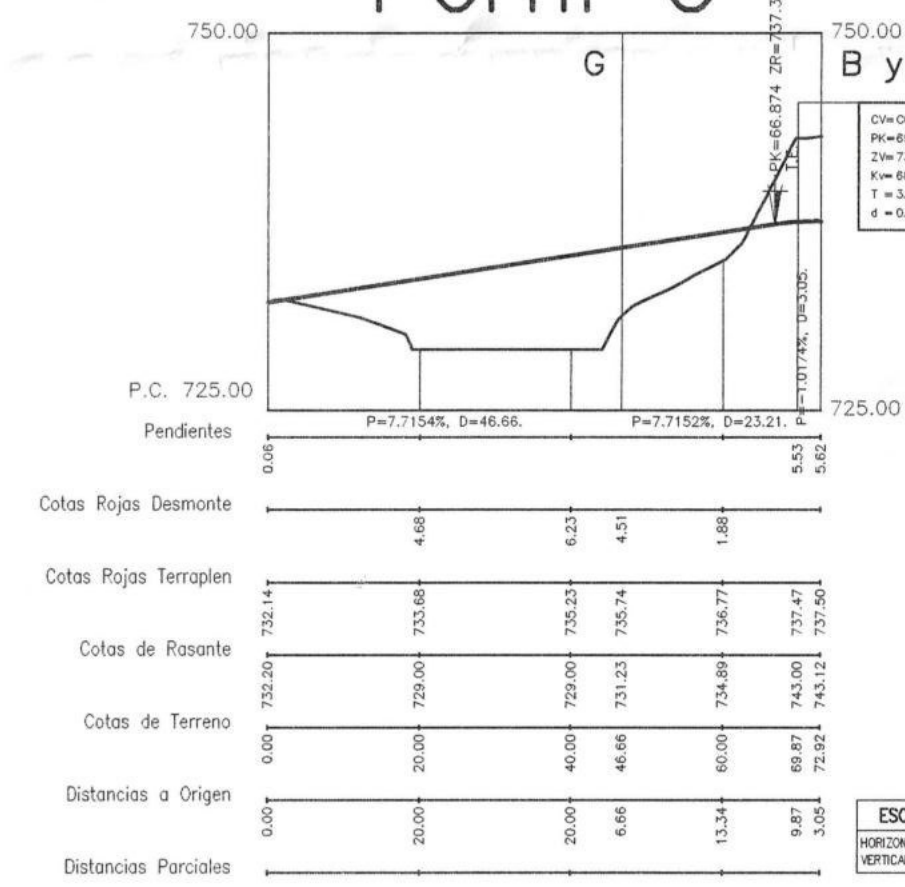
Perfil C
