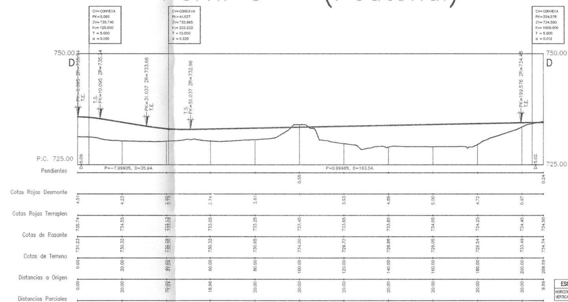
Perfil G - (Peatonal)
