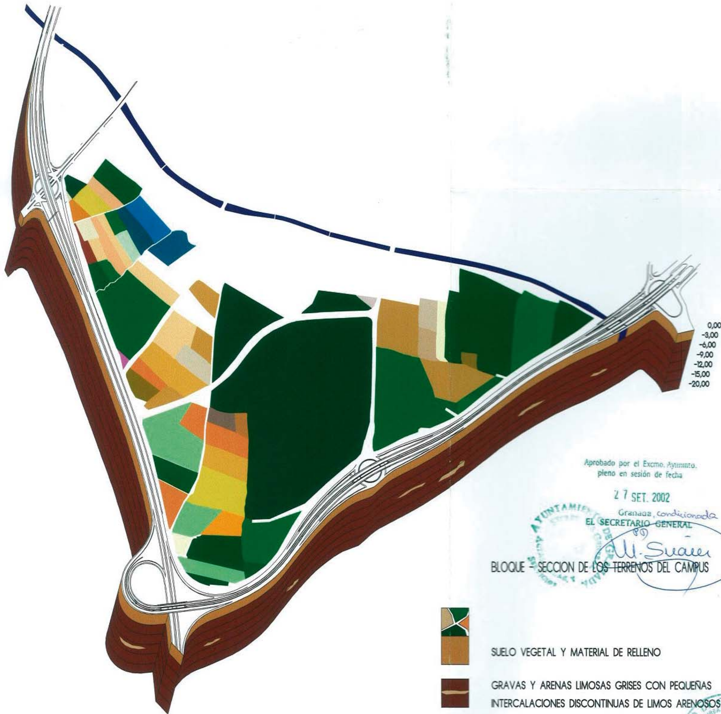
MAPA LITOLÓGICO SIMPLIFICADO.
